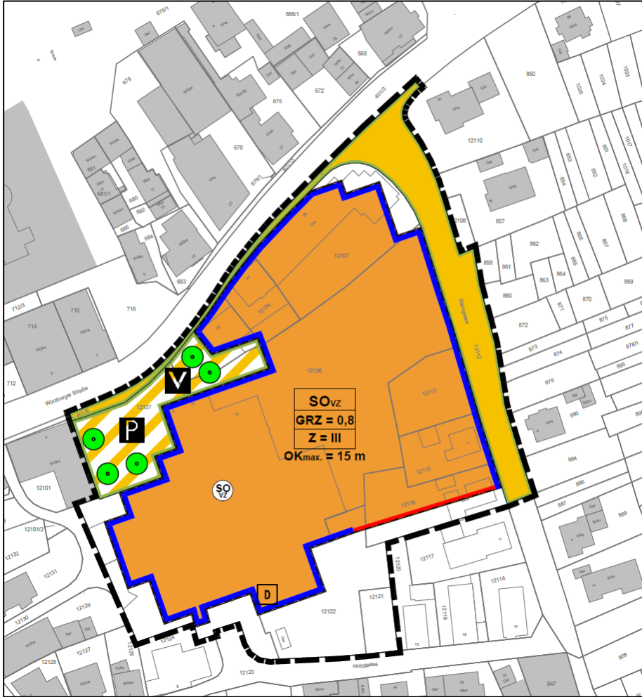
Abbildung 3: Plankarte Bebauungsplan Sanierung Hofacker B II, 1. Änderung
